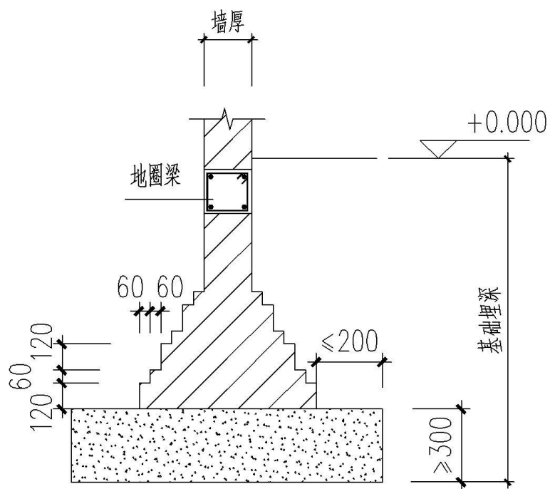
图 4-2 灰土基础剖面
