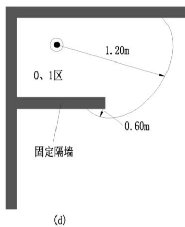
图D-2 无盆淋浴分区尺寸（二）
